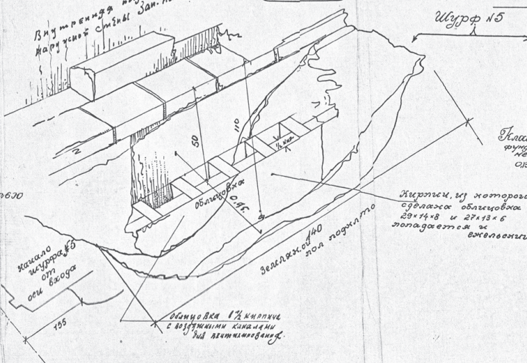
Вкладка III. Центральная проектно-реставрационная мастерская Академии Архитектуры СССР. Чертеж ЦПРМ, инв. № 1/49, 1956 г. Находится в ЦИАМ. Белокаменный Собор Андроникова монастыря. План подклета и шурфы.
