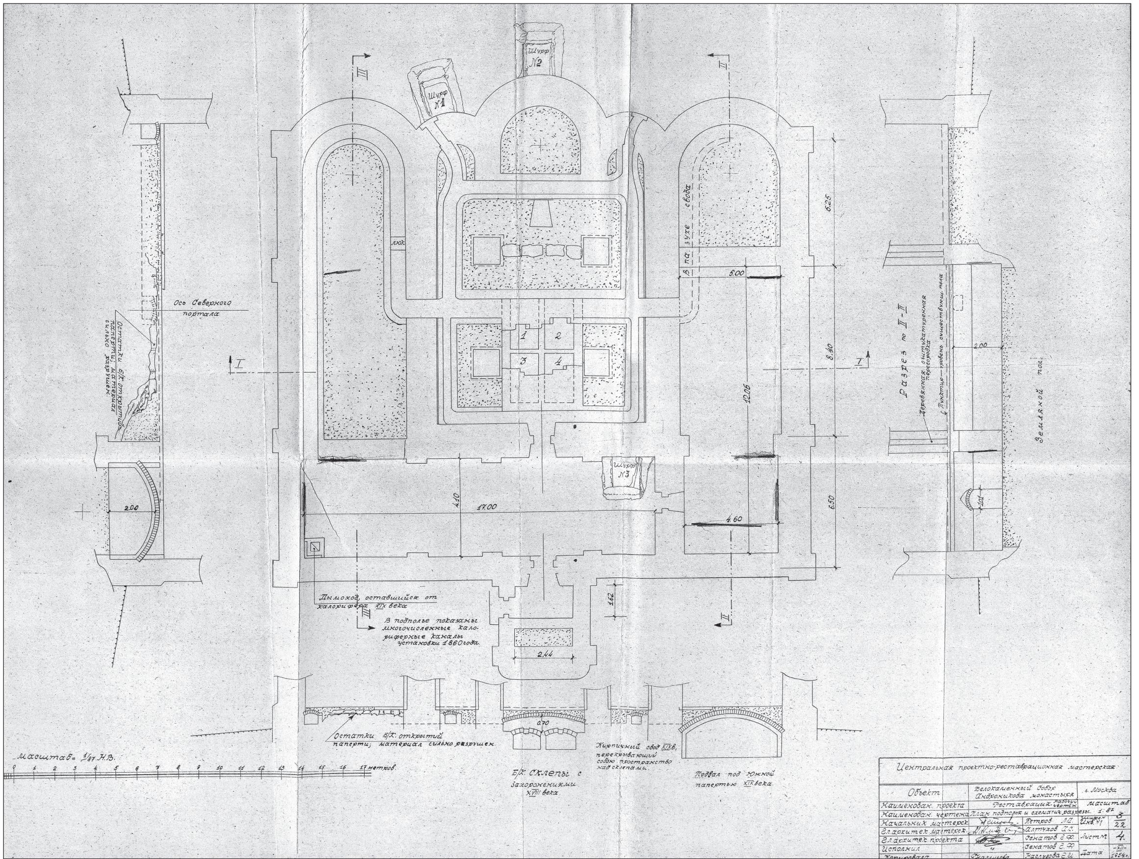
Вкладка I. Центральная проектно-реставрационная мастерская Академии Архитектуры СССР. Чертеж ЦПРМ, инв. № 3/22, 1954 г. Находится в ЦИАМ. Белокаменный Собор Андроникова монастыря. План подполья (подклета) и схематические разрезы.
