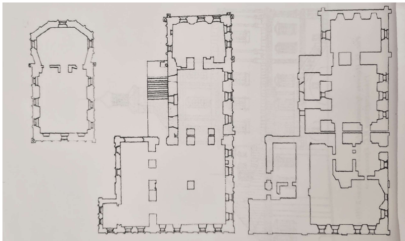
Илл. 10. Церковь Архангела Михаила (по обмерам Е. Шемруной и О. Нестеренко. 1944 г.)
