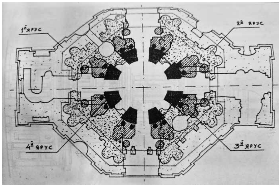
Ил. 4. Совмещенные планы ярусов колокольни конца XVIII в. Рисунок из книги И.С. Красовского «Архитектурный ансамбль Спасо-Андроникова монастыря». М., 2005. С. 127
